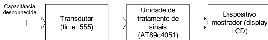
Figura 2 – Diagrama de Blocos do sistema de medição de capacitâncias.
