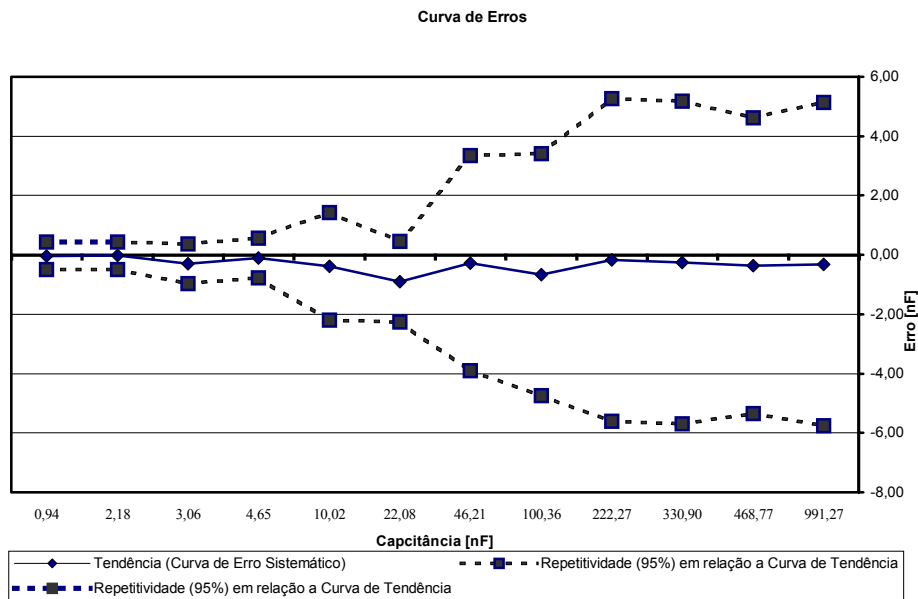
Figura 3 – Curva de erros do capacitômetro ao longo da faixa calibrada.
