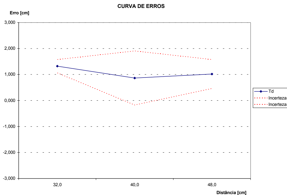
Figura 1 – Curva de erros obtida para os pontos de 32, 40 e 48 cm.
